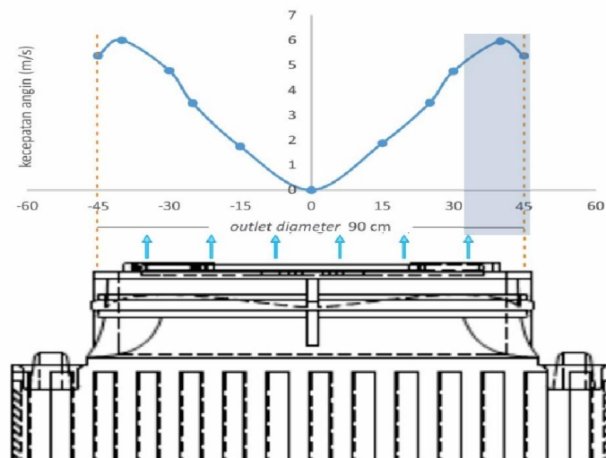
Gambar 1.1 Profil kecepatan angin yang keluar dari cooling tower
