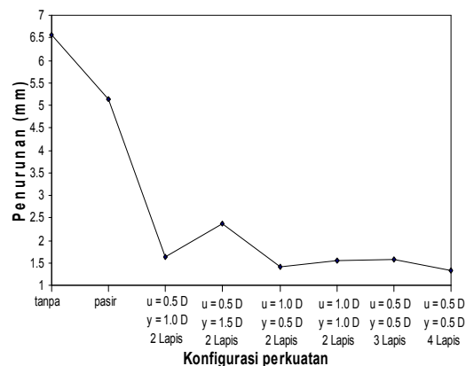
Gambar 17 Grafik hubungan penurunan dengan konfigurasi perkuatan pasir 1.0D (D=diameter pondasi) dan anyaman bambu terletak pada lapisan pasir dan tanah kohesif pada beban 200 Kgf
