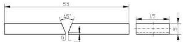
Gambar 10. Bentuk Kampuh Las pada Spesimen 2
