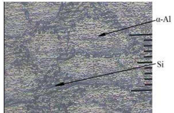
Gambar 12. Struktur Mikro Logam Dasar ( Raw material )
