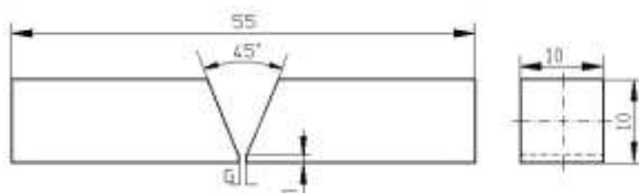
Gambar 8. Bentuk Kampuh Las pada Spesimen 1
